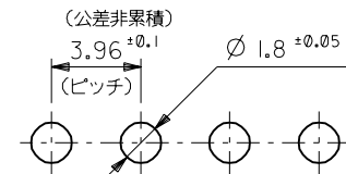
基板取付穴推奨寸法
