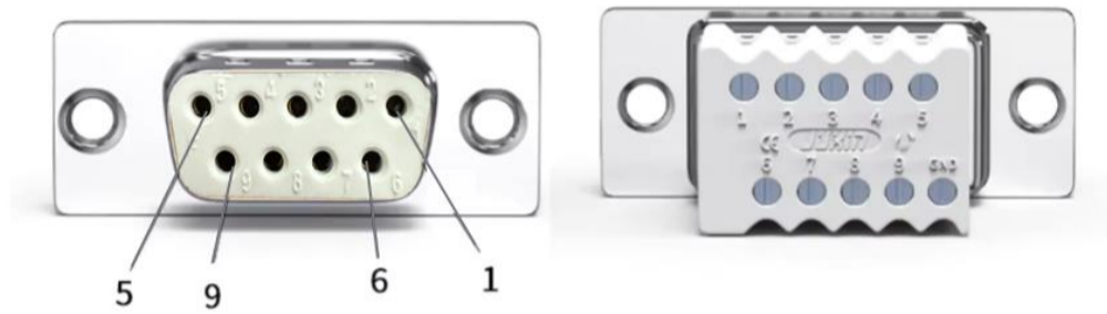
DB9 무납땜 커넥터(Female) 핀맵
