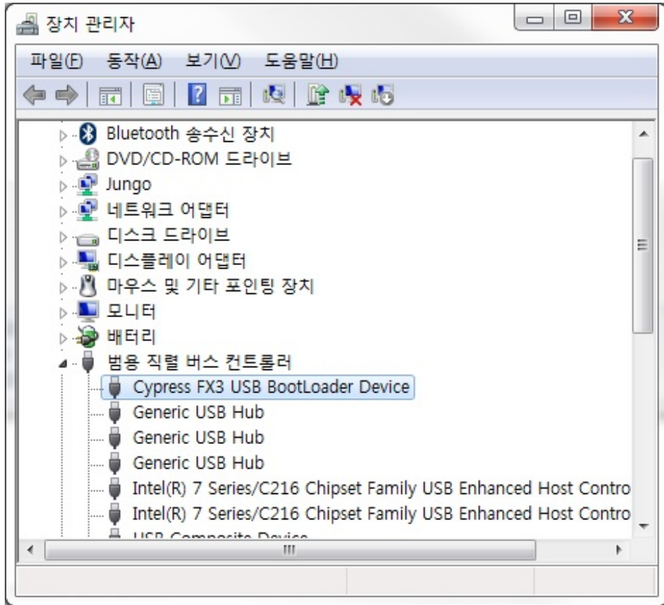
그림 3. 드라이버 설치
