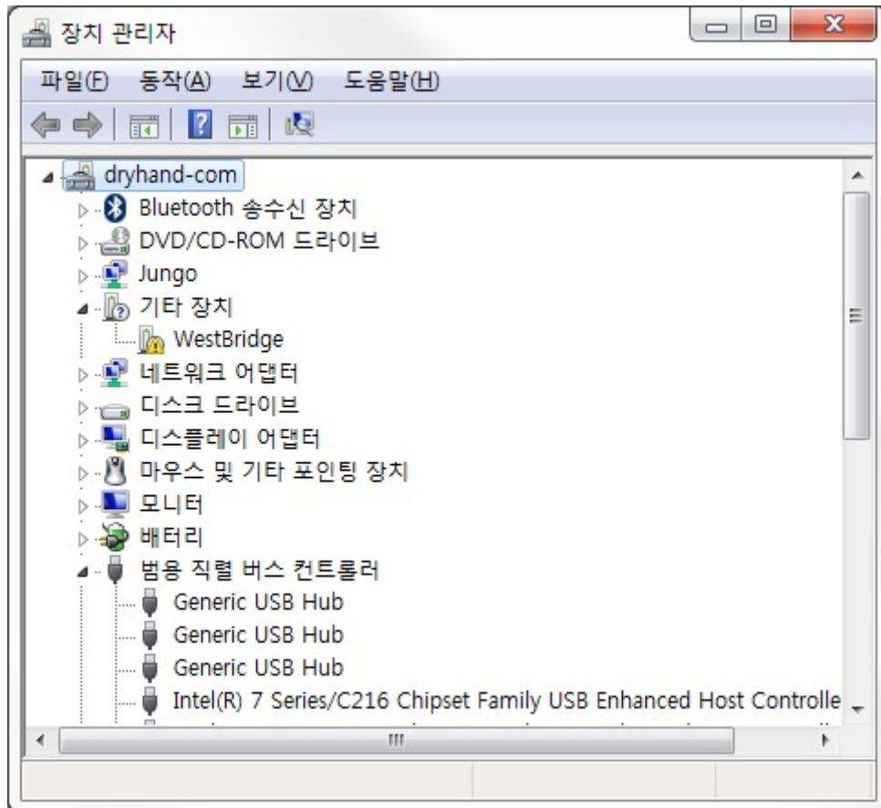
그림 2. 디바이스 변경
